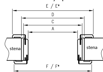
Horizontálny #prierez
