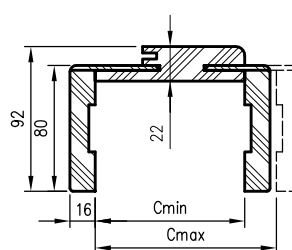
Prierez ORB
