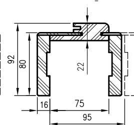
Prierez ORB_075
