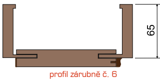
profil zárubně č. 6
