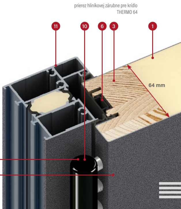
prierez ocelevej zárubne pre krídlo THERMO 64
