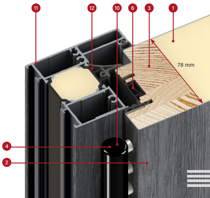
prierez hliníkovej zárubne pre krídlo THERMO HOT 78
